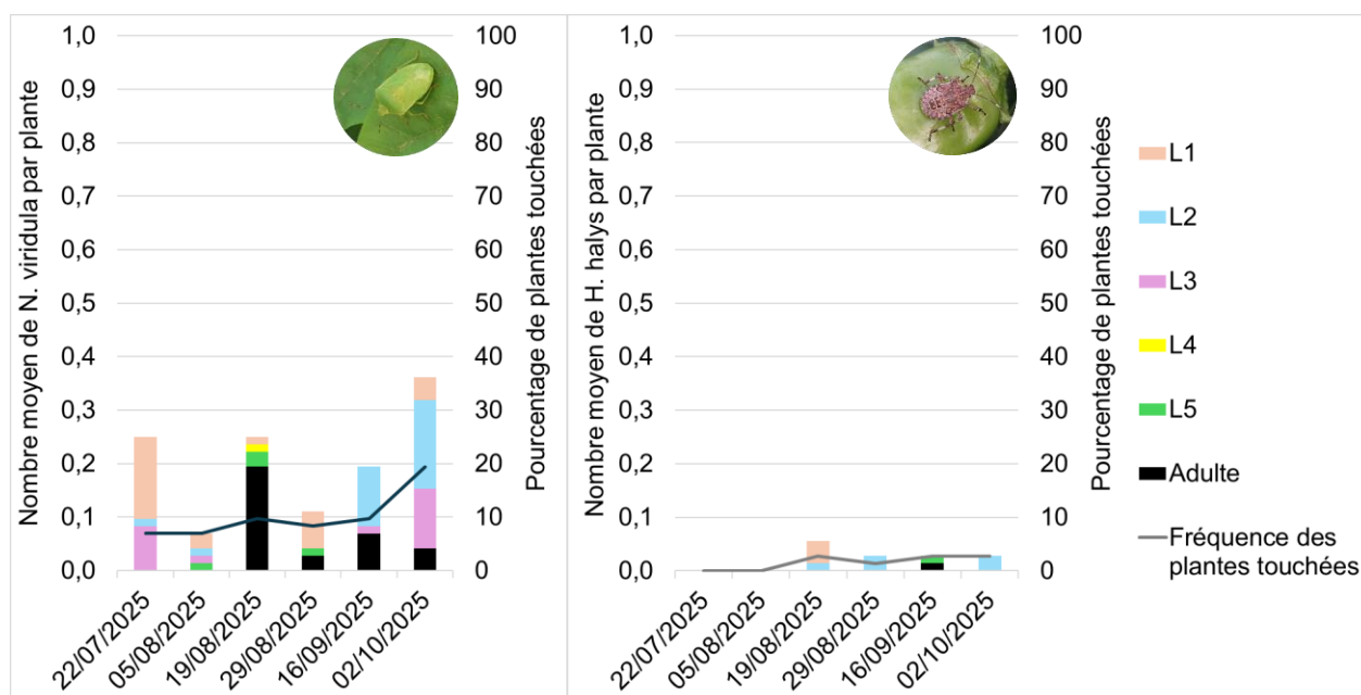
Figure 20 : Dynamique de population des punaises Nezara viridula (graphique de gauche) et de Halyomorpha halys (graphique de droite), effectifs moyens des différents stades de punaises et fréquence de plantes touchées
